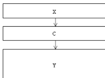
Gambar 2. Kerangka Analisis
